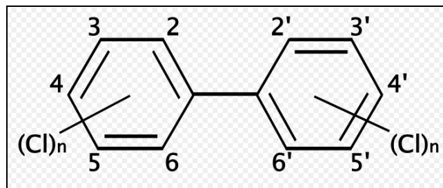
Figura 1 – Estrutura molecular dos PCB
